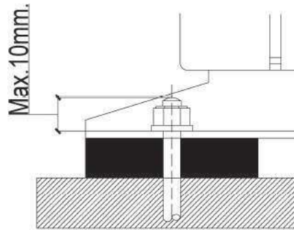
Αντικραδασμικό λάστιχο
